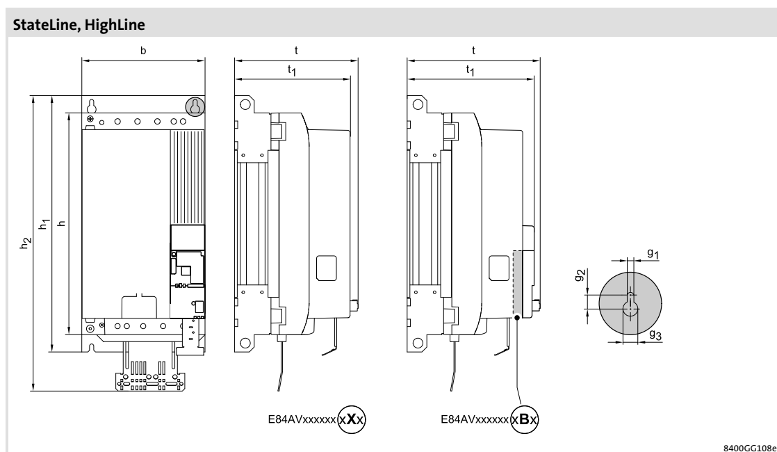
rys. 5-41 Wymiary urządzeń
