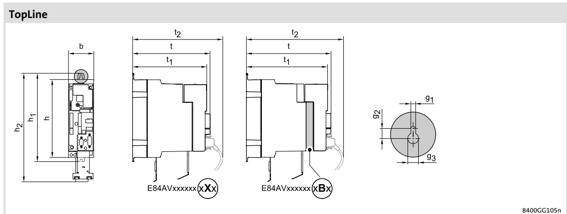
rys. 5-3 Wymiary urządzeń
