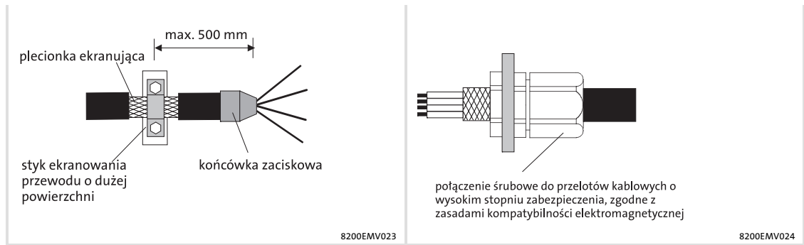
rys. 6-3 Ekranowanie przewodu silnika
