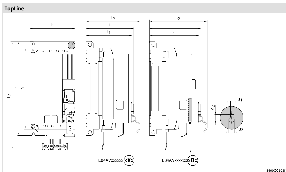
rys. 5-43 Wymiary urządzeń
