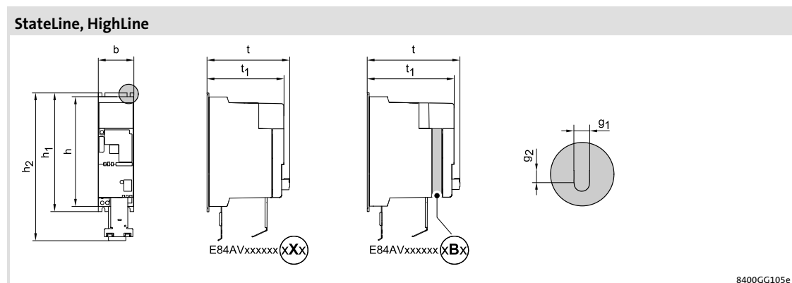
rys. 5-15 Wymiary urządzeń
