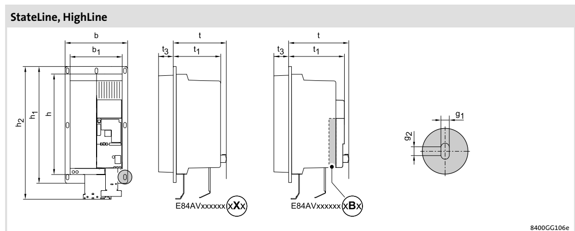
rys. 5-25 Wymiary urządzeń
