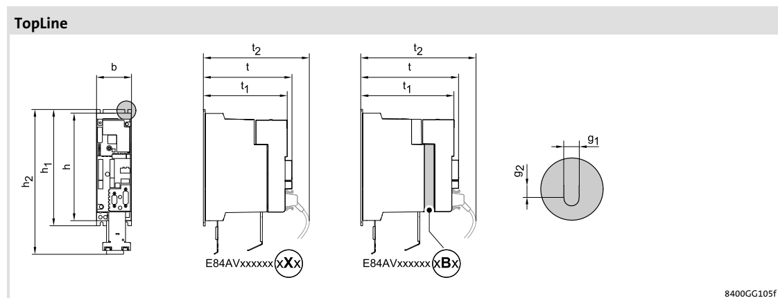
rys. 5-17 Wymiary urządzeń
