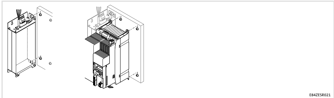
rys. 5-24 Montaż z filtrem montowanym z boku
