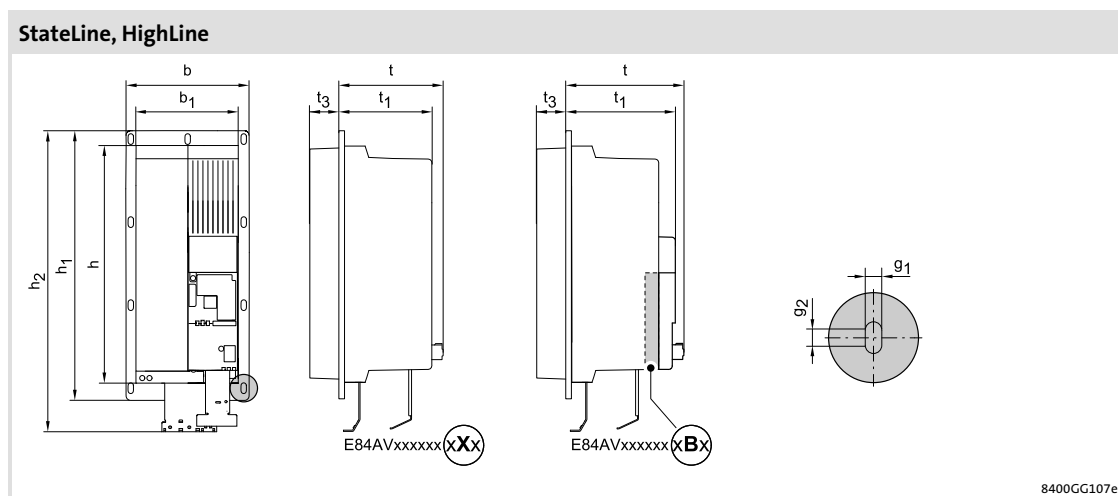
rys. 5-29 Wymiary urządzeń
