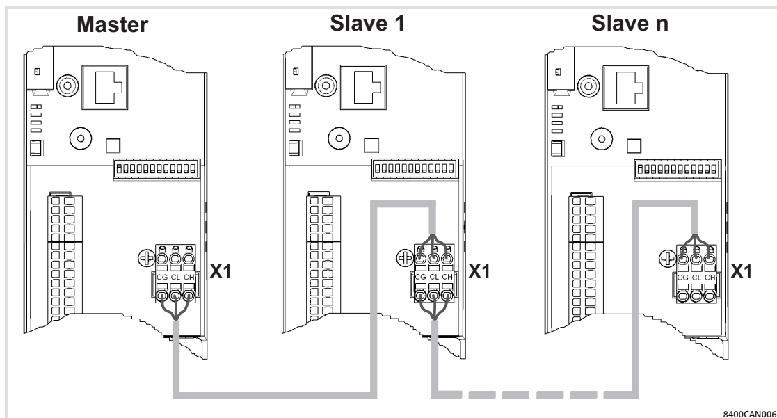
rys. 6-31 Okablowanie magistrali systemowej (CAN)
