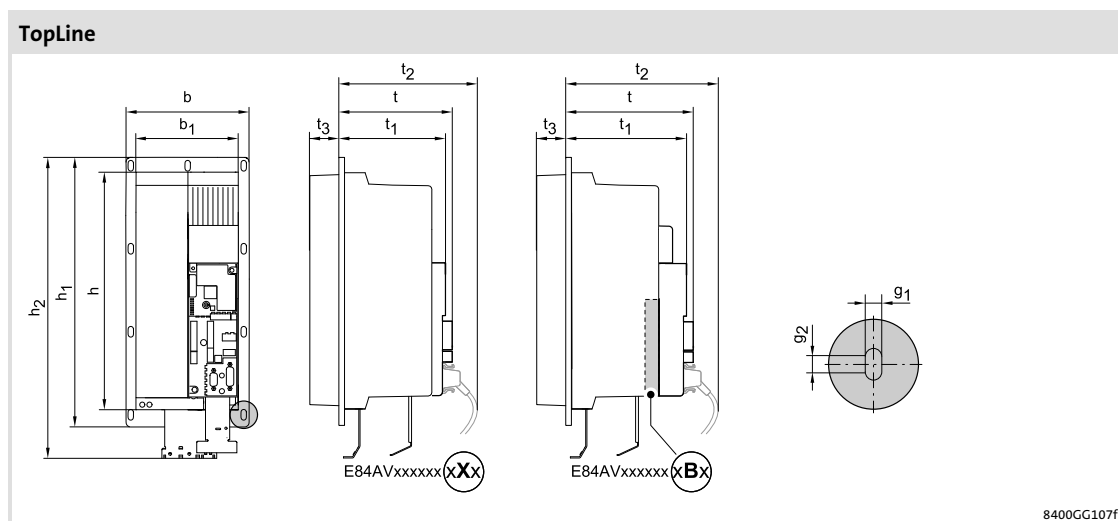
rys. 5-31 Wymiary urządzeń
