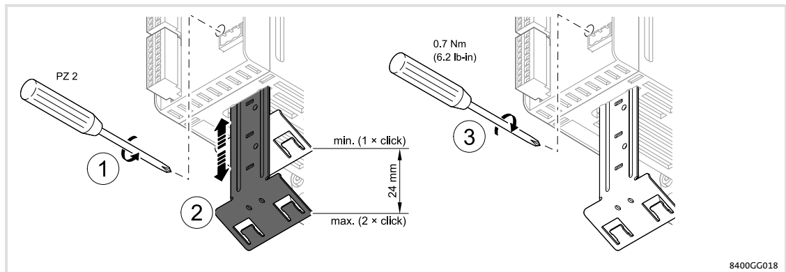
rys. 6-25 Mocowanie płytki ekranującej
