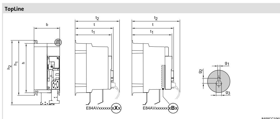
rys. 5-21 Wymiary urządzeń
