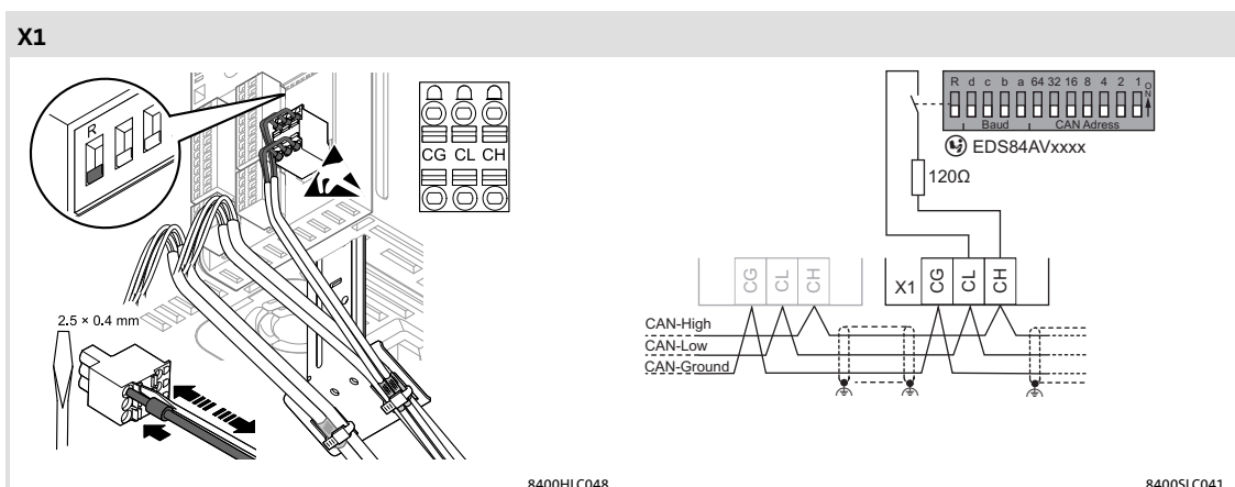
rys. 6-29 Podłączenie CANopen
