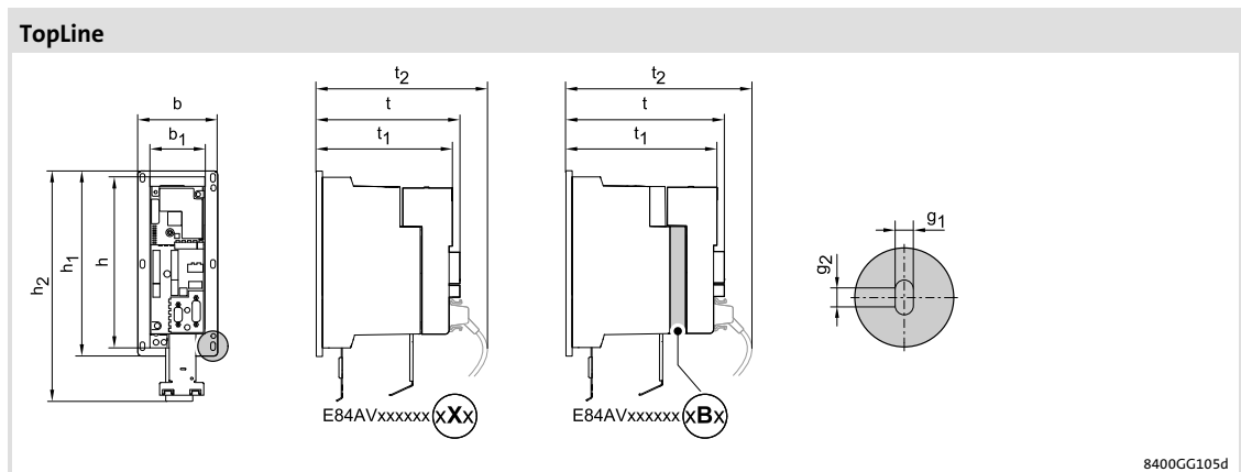
rys. 5-13 Wymiary urządzeń
