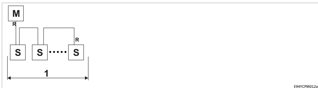
rys. 6-27 Przykład: sieć CAN z jednym segmentem
