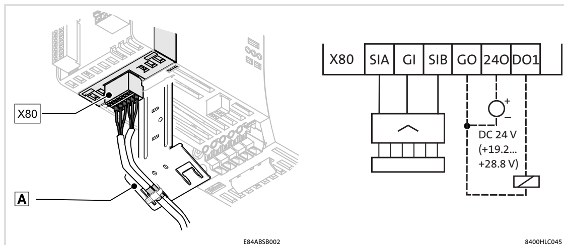
rys. 10-2 Schemat ideowy połączeń układu zabezpieczającego (STO)
