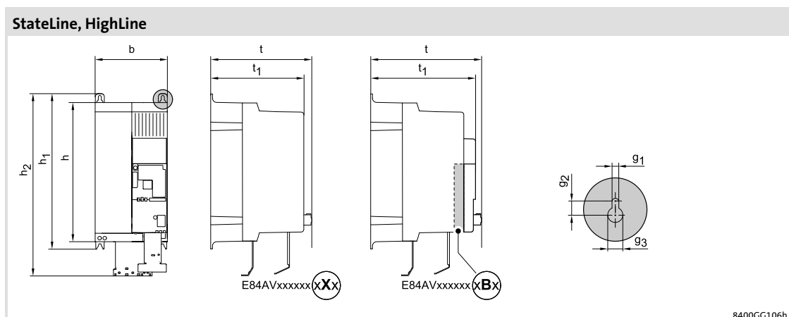
rys. 5-19 Wymiary urządzeń
