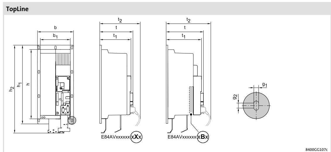
rys. 5-39 Wymiary urządzeń
