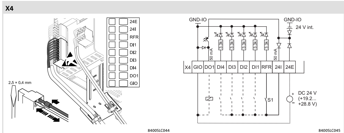
rys. 6-33 Podłączenie do zewnętrznego napięcia zasilającego
