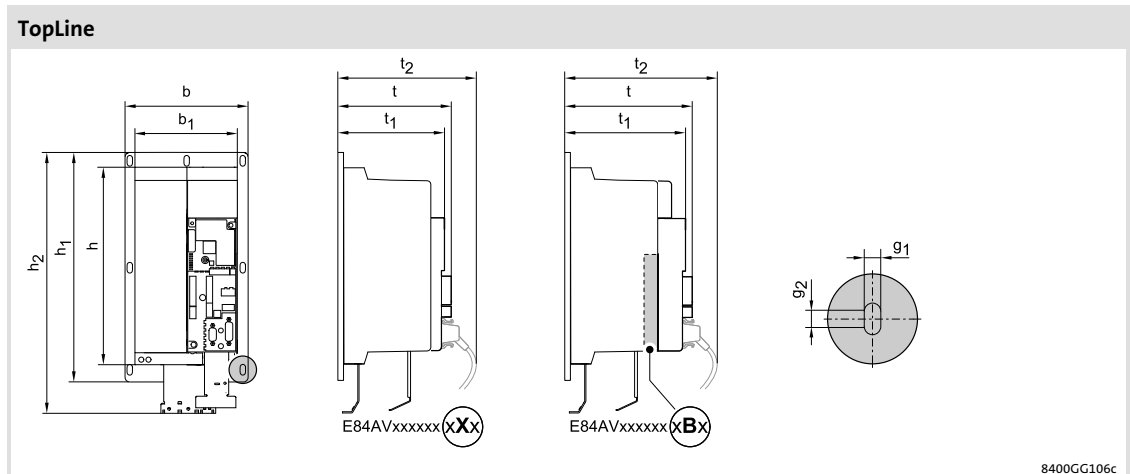
rys. 5-35 Wymiary urządzeń
