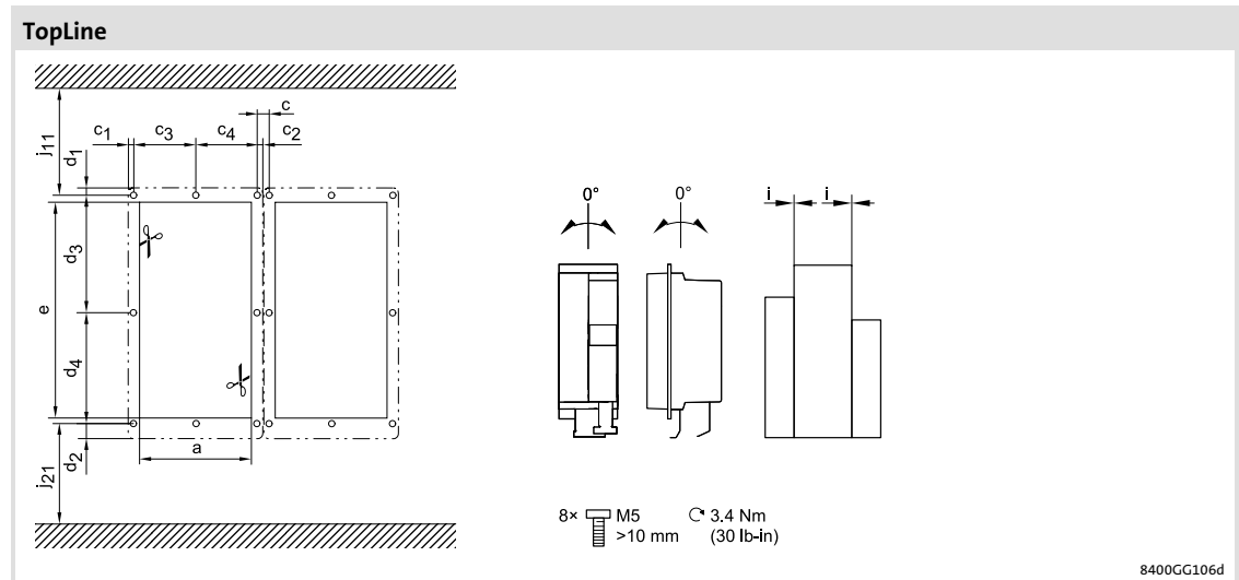
rys. 5-28 Wymiary do montażu
