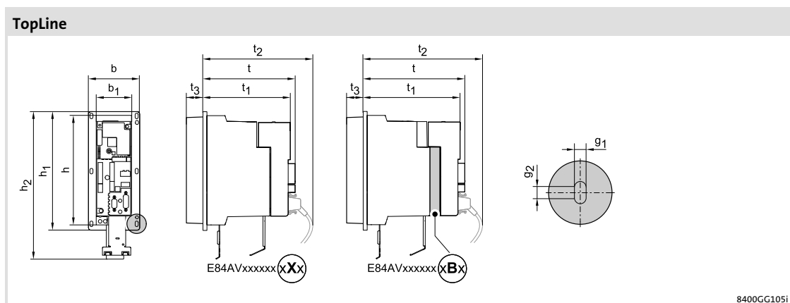
rys. 5-9 Wymiary urządzeń
