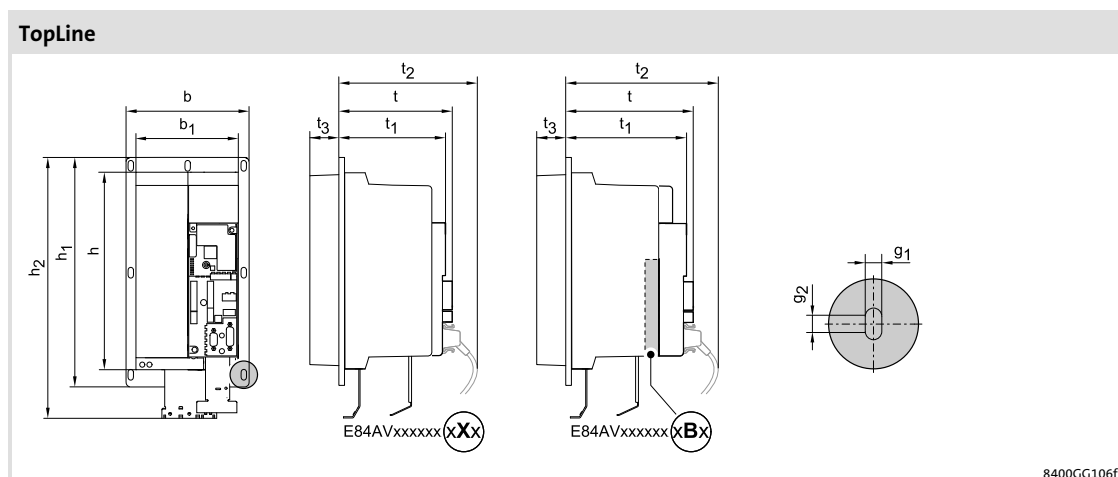
rys. 5-27 Wymiary urządzeń
