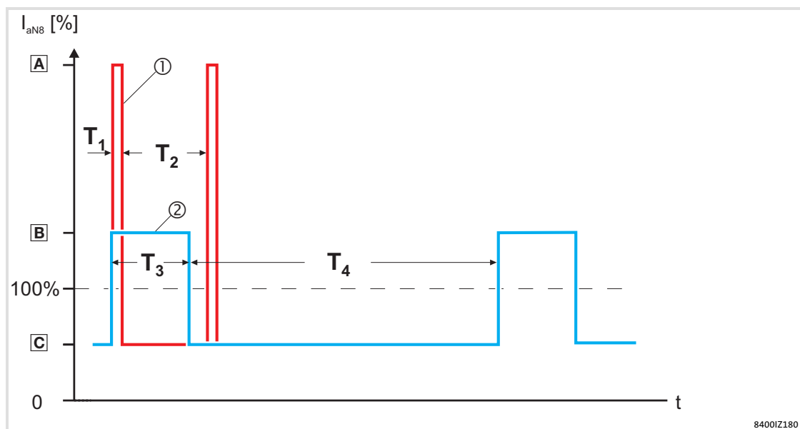
rys. 4-2 Zdolność przeciążania w pracy z 230/400 V przy 45° C
