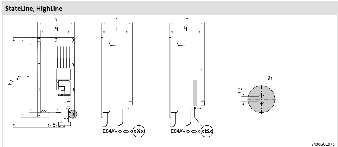
rys. 5-37 Wymiary urządzeń
