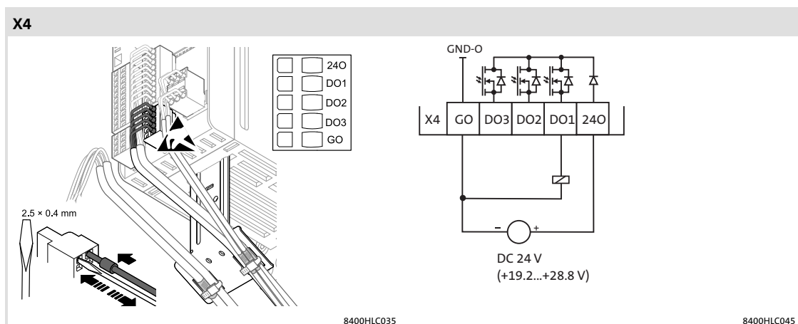
rys. 6-43 Podłączenie wyjść cyfrowych
