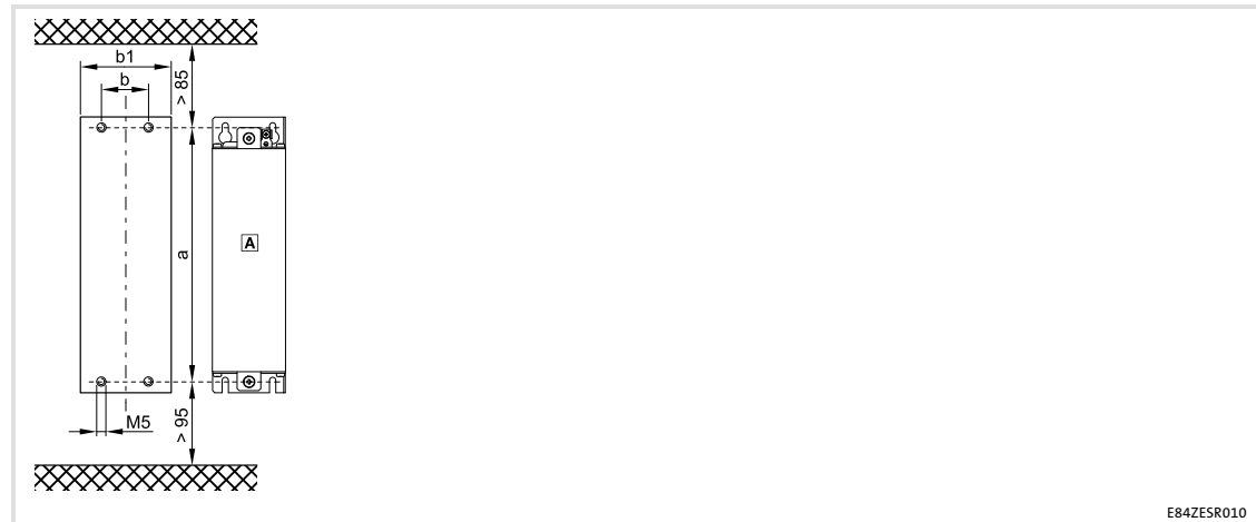
A Filtr montowany pod spodem
