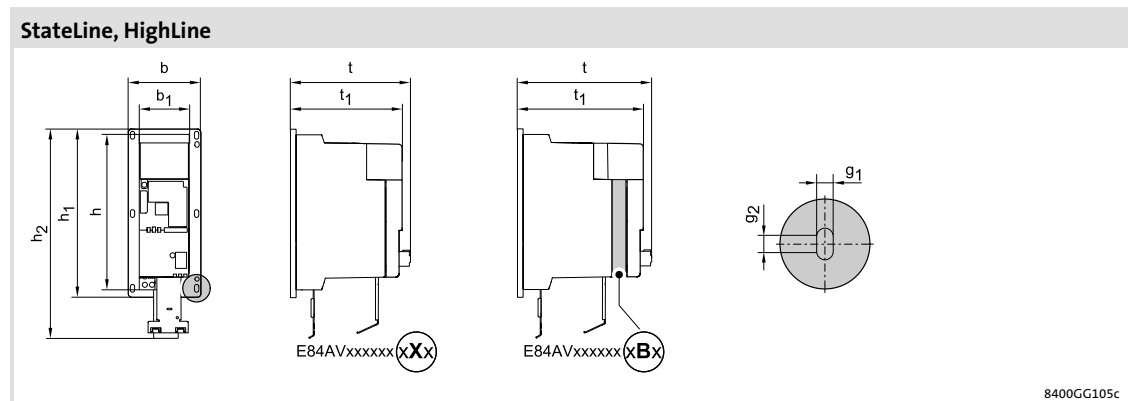
rys. 5-11 Wymiary urządzeń
