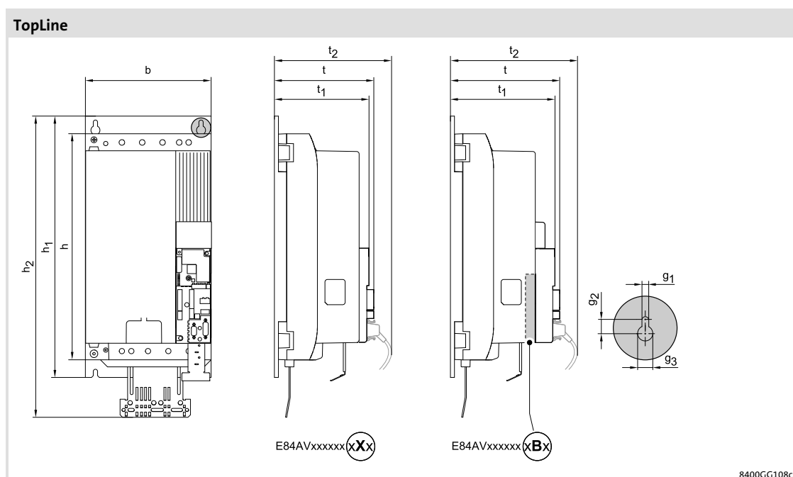
rys. 5-47 Wymiary urządzeń
