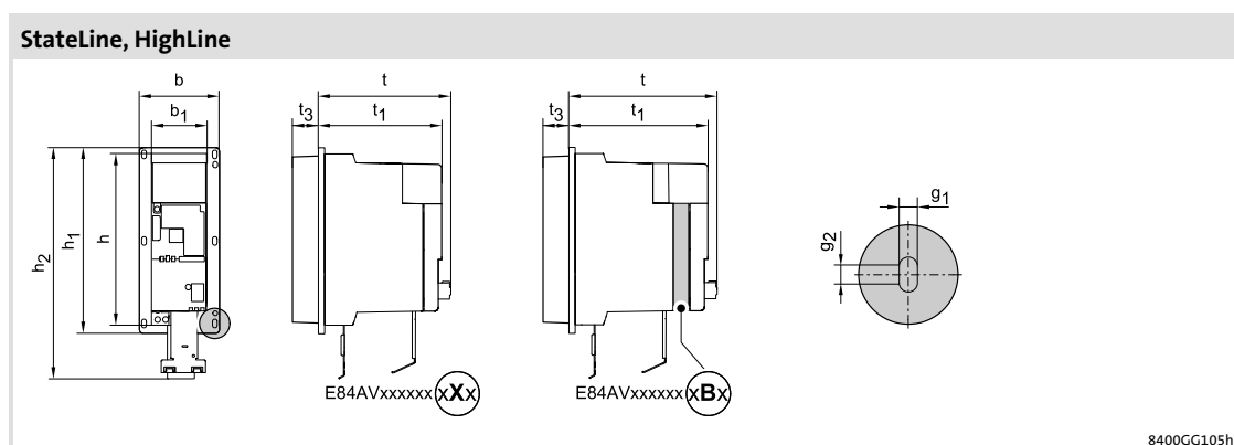
rys. 5-7 Wymiary urządzeń
