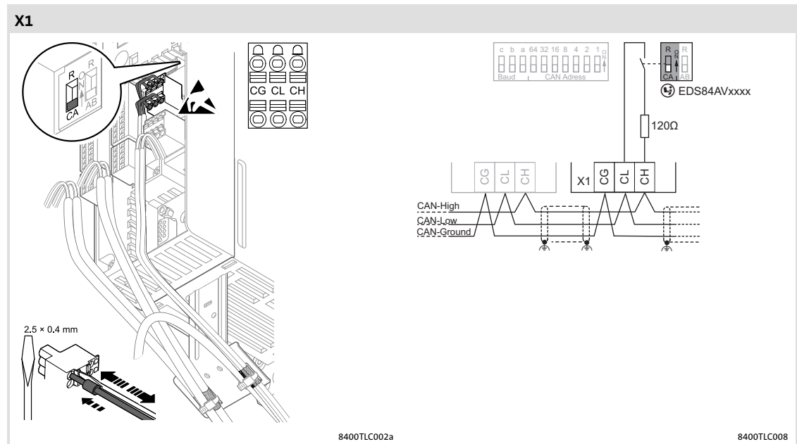
rys. 6-30 Podłączenie CANopen
