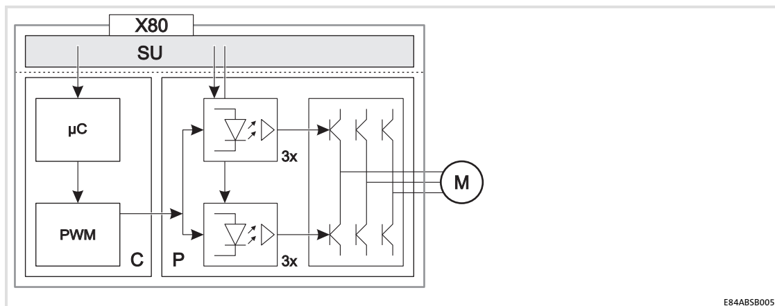
rys. 10-1 Zasada działania układu technologii bezpieczeństwa
