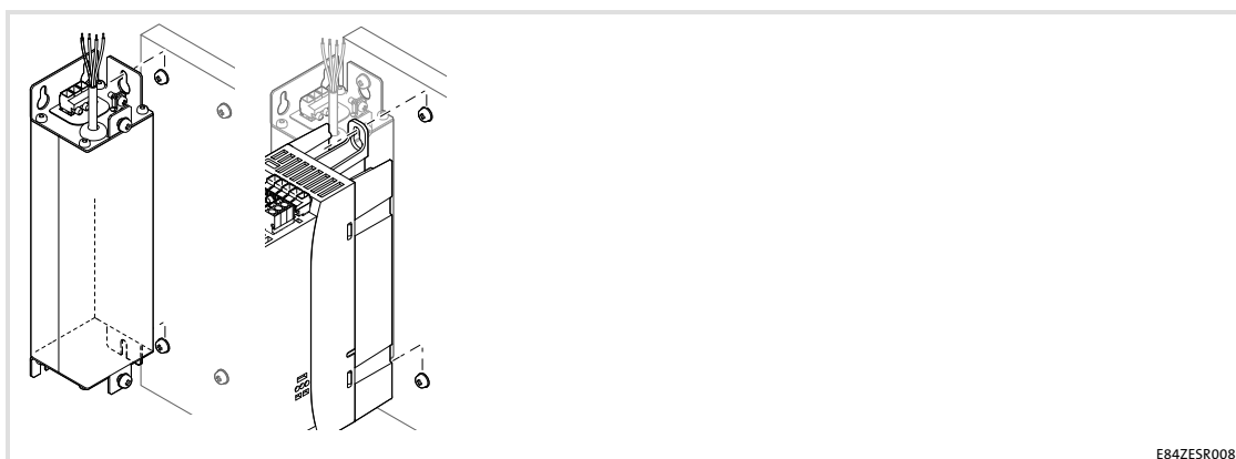
rys. 5-6 Montaż z filtrem montowanym z boku
