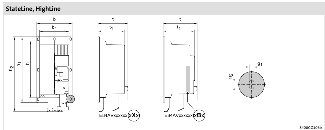
rys. 5-33 Wymiary urządzeń
